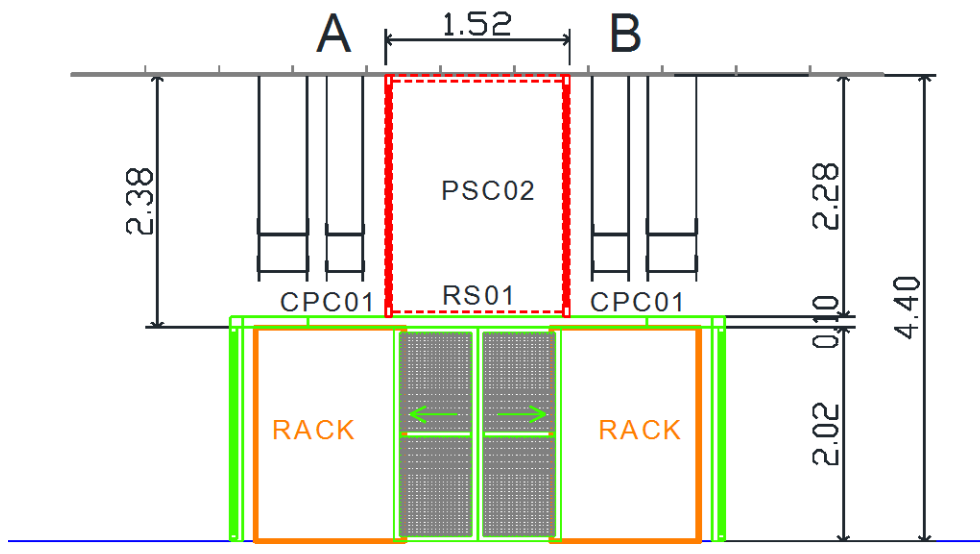
Elevacion - Barrera Perimetral
