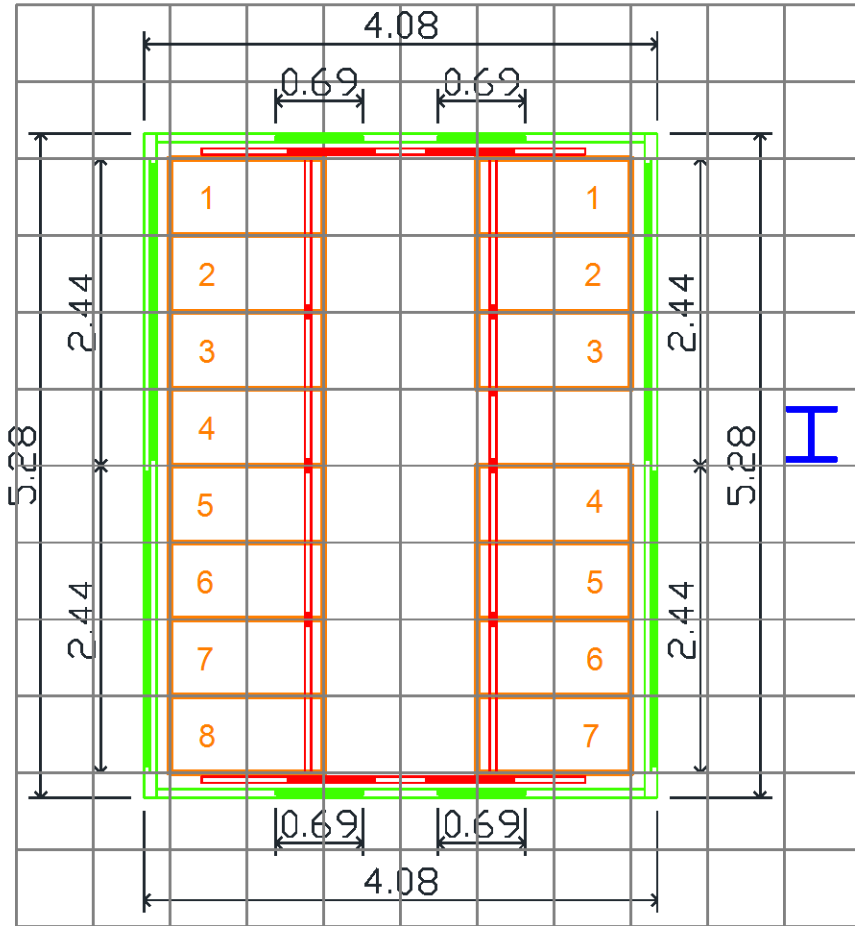
Planta - Barrera Perimetral
