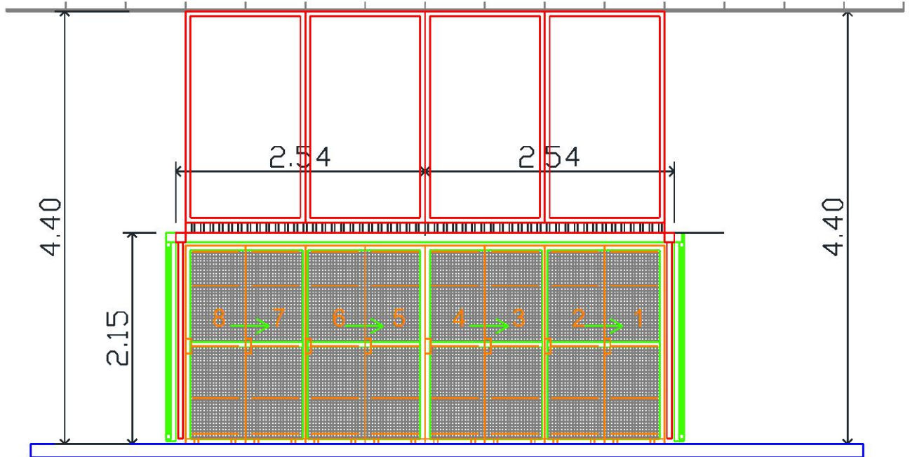
Elevacion - Barrera Perimetral
